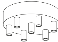
KRM576FVBOTERM 7 HOLE Ø 120MM H 25MM
